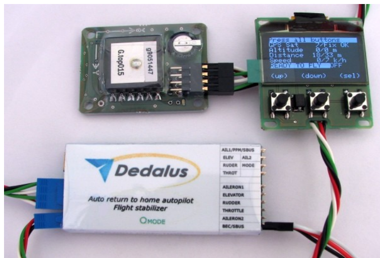
Рис. 1 Комплект автопилота
