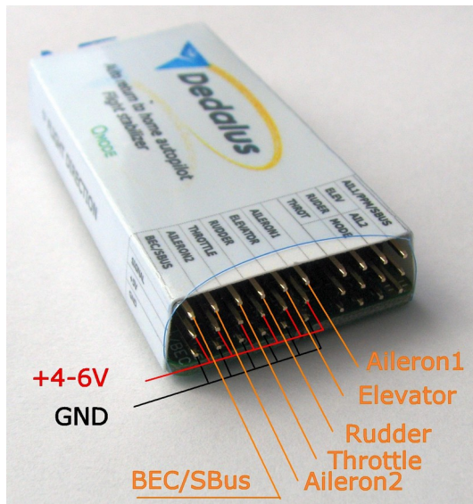
Рис. 4 Выходы автопилота
